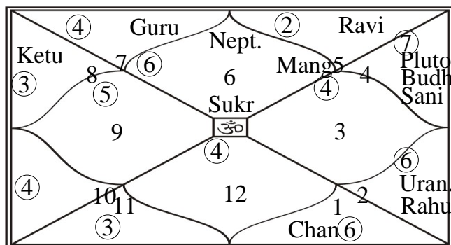
Sukr
