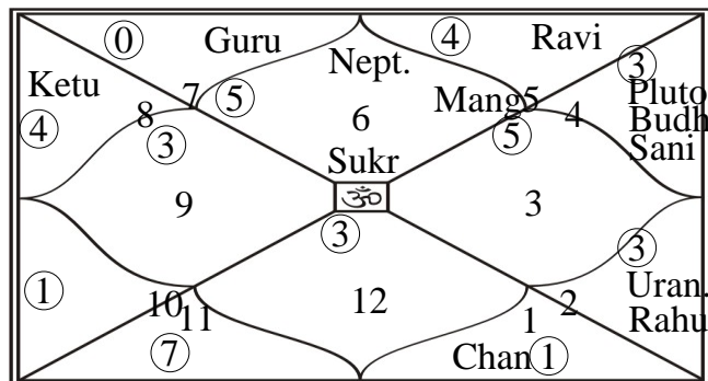
Sani
